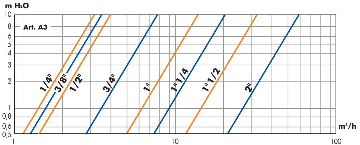
Diagramma perdita di carico. Fluido: H 2 O - Loss of head diagram. Fluid: H 2 O
